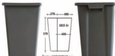
TRP-KÜFE-9 370*480*570 MM
